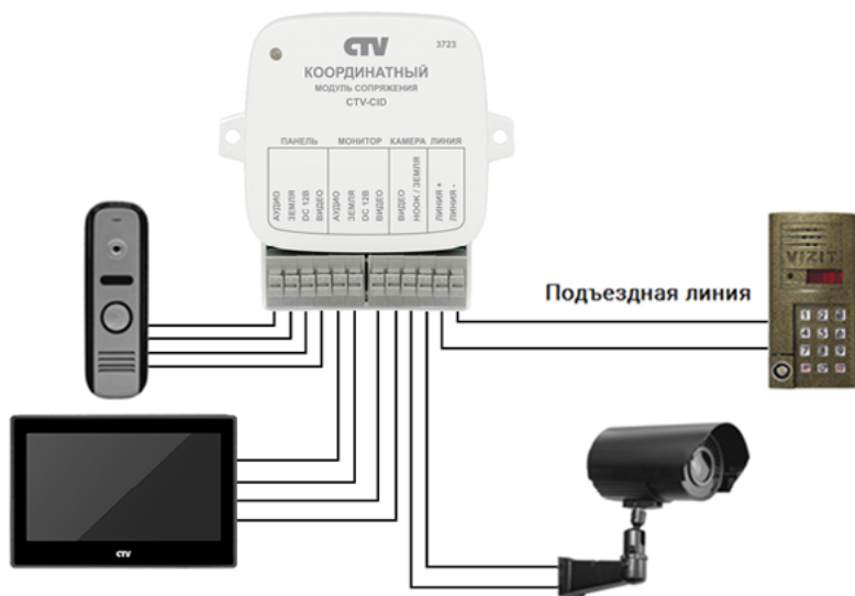
Рисунок 3 — Подключение компонентов домофонной системы
