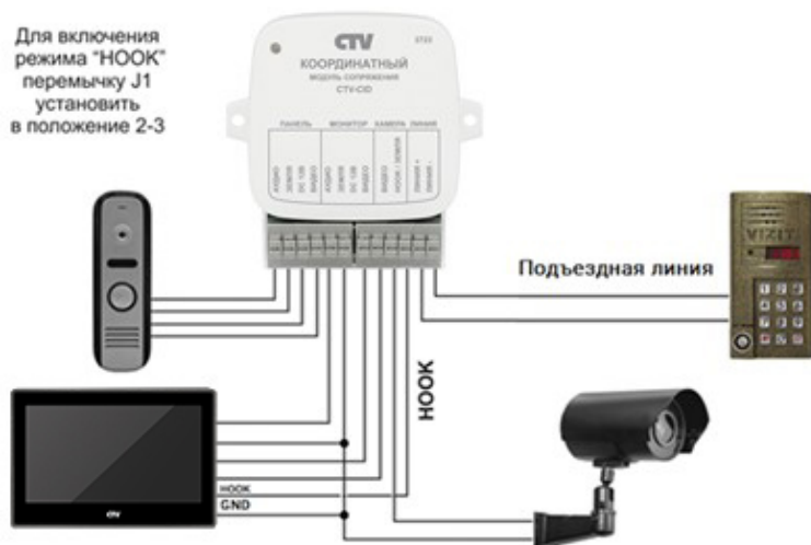
Рисунок 4 – Использование сигнала НООК
